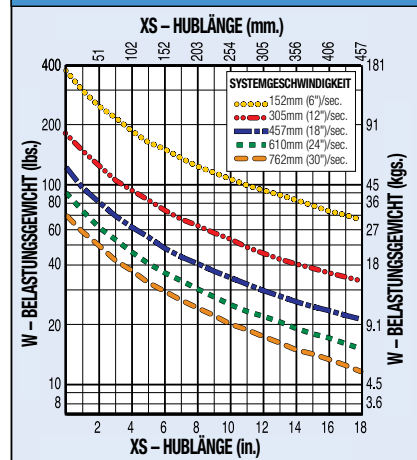
MAXIMALES LASTGEWICHT ZUR HUBLÄNGE VERBUNDLAGER, ÜBERDIMENSIONIERTE FÜHRUNGSSTÄBE
