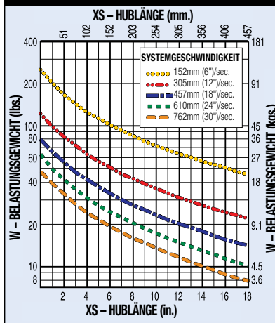
MAXIMALES LASTGEWICHT ZUR HUBLÄNGE VERBUNDLAGER, STANDARD-FÜHRUNGSSTANGEN
