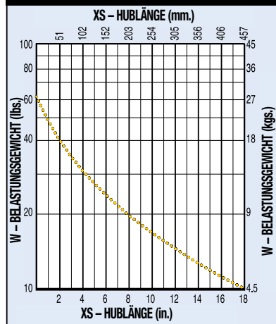
MAXIMALES LASTGEWICHT ZUR HUBLÄNGE LINEARKUGELLAGER, STANDARD-FÜHRUNGSSTANGEN
