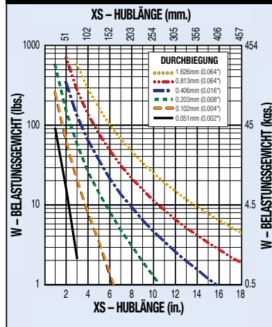
DURCHBIEGUNG DER FÜHRUNGSSTANGE STANDARD-FÜHRUNGSSTANGE
