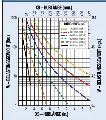
DURCHBIEGUNG DER FÜHRUNGSSTANGE ÜBERDIMENSIONIERTE FÜHRUNGSSTÄBE
